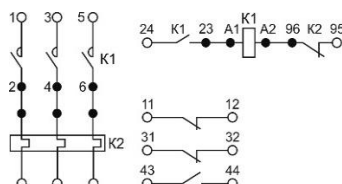
Рисунок 6. Пускатель серии ПМА нереверсивный без реле
