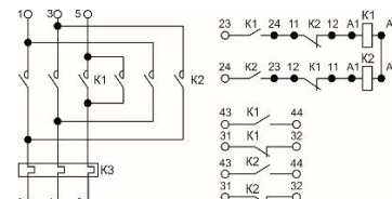
Рисунок 7. Пускатель серии ПМА реверсивный без реле
