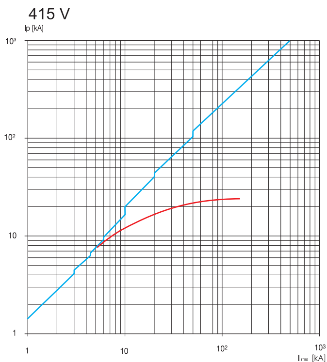
MNX250 Кривая ограничения тока
