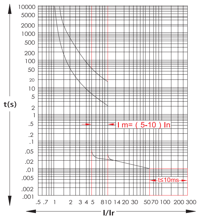
MNX160 - TMD
