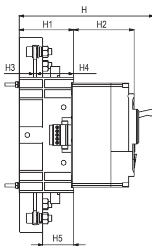
Фронтальное подключение
