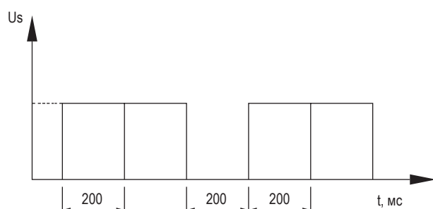
Схема работы SHT 125-630AF
