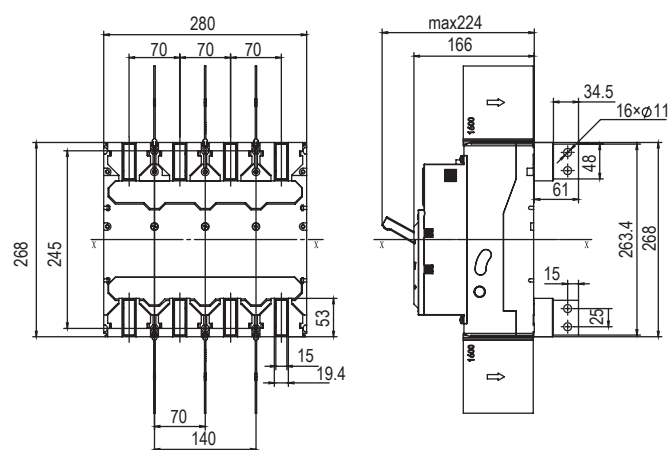
MNX1600 вертикальное заднее подключение
