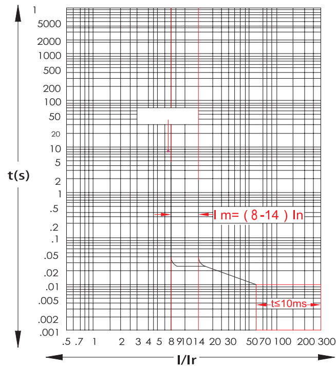
MNX160 - TMM
