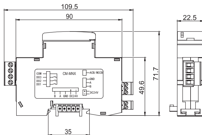
Размеры
