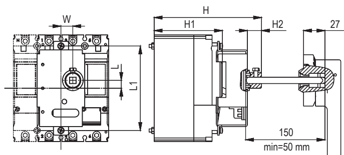
Монтажные размеры
