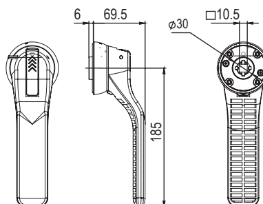
Вырез в двери шкафа MNX1600
