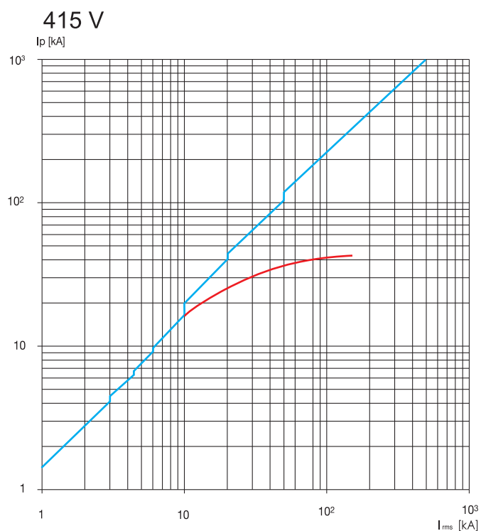
MNX630 Кривая ограничения тока
