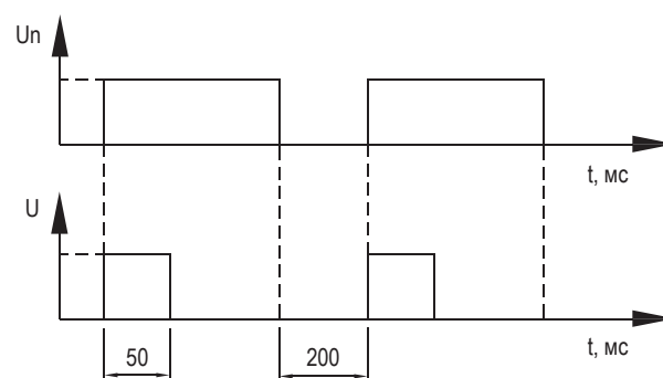
Схема работы SHT 125-630AF
