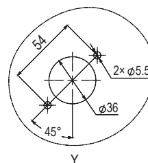
Вырез в двери шкафа
