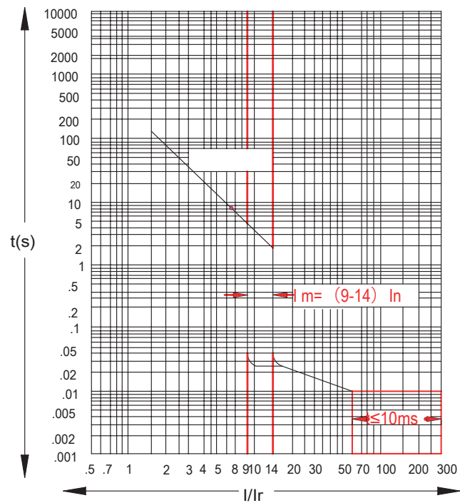
MNX250 - TMM
