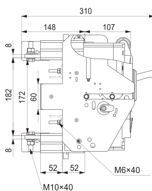
Заднее подключение
