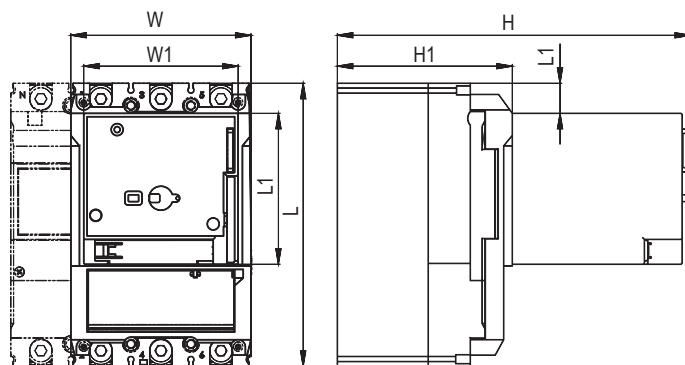
Габаритные размеры
