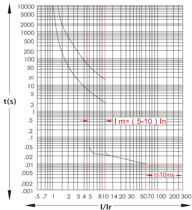
MNX125 - TMD
