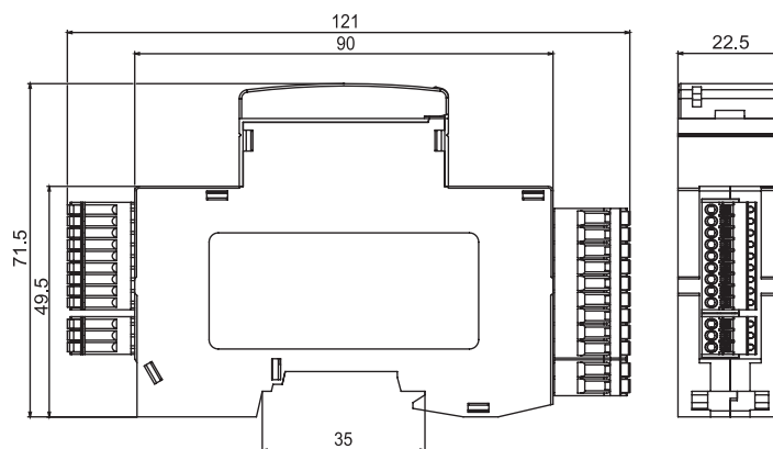
Размеры
