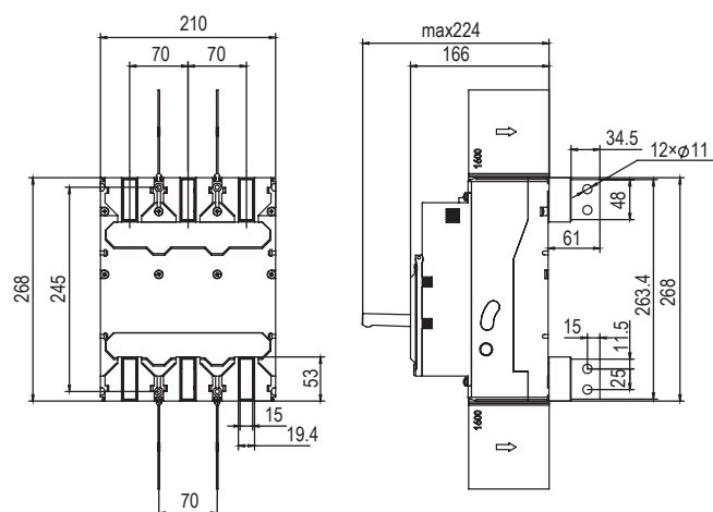
MNX1600 вертикальное заднее подключение
