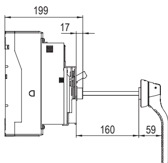
Монтажные размеры MNX1600
