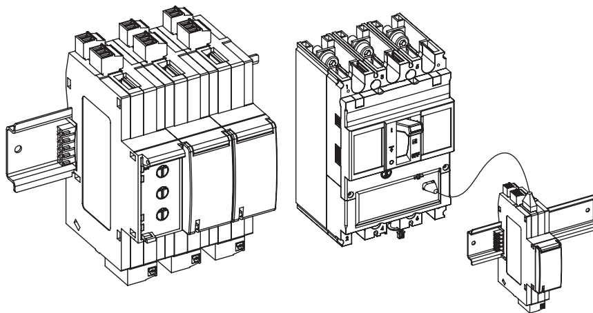
Установка на DIN рейку
