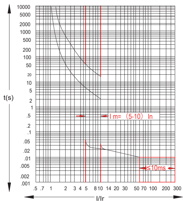
MNX250 - TMD
