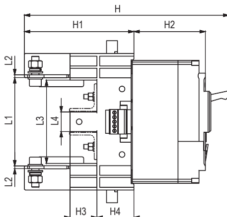
Заднее подключение
