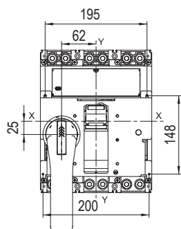
Монтажные размеры MNX1600
