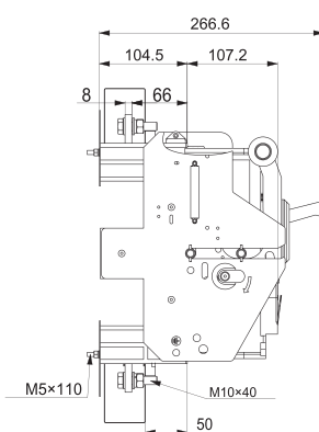
Фронтальное подключение
