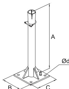
Подставка 5–7 метров
