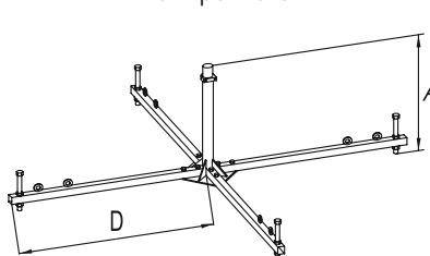
Четырёхнога
