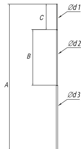
Мачты 8–10 метров
