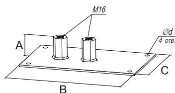
Подставка 1–4 метра
