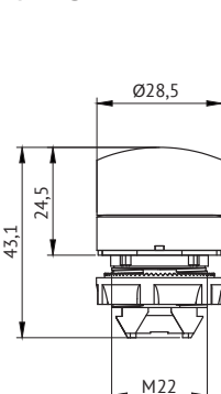
Головка переключателя OptiSignal D22 A5-S и головка переключателя с подсветкой OptiSignal D22 A5-SL
