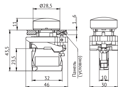
Лампа сигнальная OptiSignal D22 C4-L
