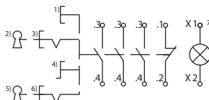
Выключатели/переключатели с тремя замыкающими и одним размыкающим контактами
