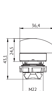
Головка переключателя с удлиненной ручкой OptiSignal D22 A5-SJ
