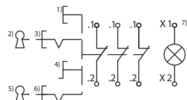
Выключатели/переключатели с тремя замыкающими контактами
