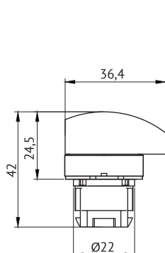
Головка переключателя с удлиненной ручкой OptiSignal D22 A4-SJ
