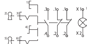
Выключатели/переключатели с одним замыкающим и двумя размыкающими контактами
