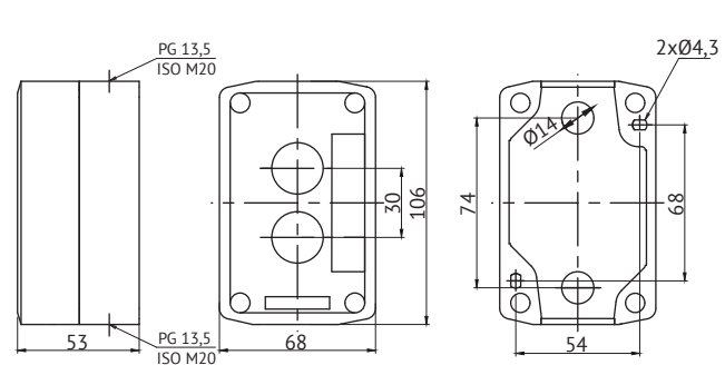
Посты OptiSignal D22 A5-BD-2
