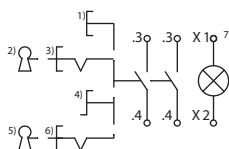
Выключатели/переключатели с двумя замыкающими контактами
