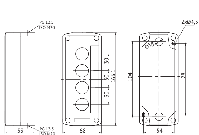
Посты OptiSignal D22 A5-BD-4
