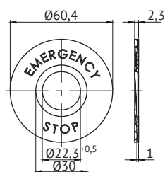
Табличка с маркировкой «Emergency stop» OptiSignal D22 A45-MH2560
