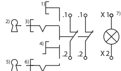
Выключатели/переключатели с двумя замыкающими контактами
