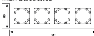
РАМКА ЧЕТЫРЕХМЕСТНАЯ
