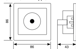
РОЗЕТКА ТЕЛЕВИЗИОННАЯ, КОМПЬЮТЕРНАЯ, КОМПЬЮТЕРНАЯ ДВОЙНАЯ
