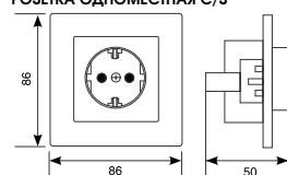
РОЗЕТКА ОДНОМЕСТНАЯ С ПРОЗРАЧНОЙ КРЫШКОЙ С/З
